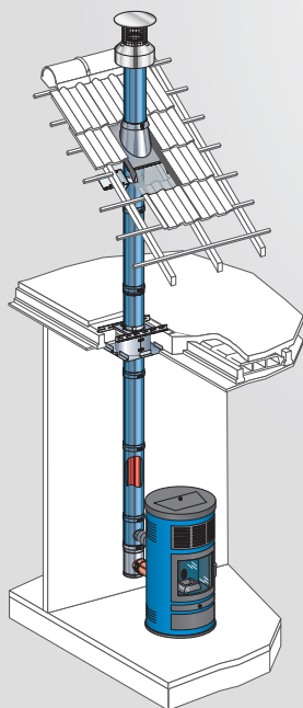
Ortakinis-dūmtakinis dūmtraukis BI-PELLET; prijungimas (BI-PELLET)
