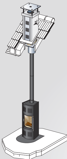
Izoliuotas dūmtraukis DUALINOX; prijungimas (STARTINOX)
