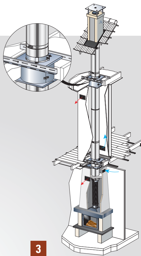
Izoliuotas dūmtraukis DUALINOX; prijungimas (STARFLEX KIT I)
