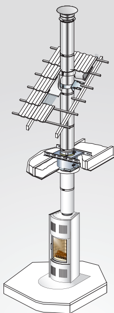
Izoliuotas dūmtraukis DUALINOX; prijungimas (DUALINOX)
