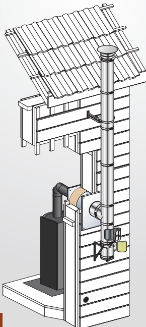
Izoliuotas dūmtraukis DUALINOX; prijungimas (DUALINOX)
