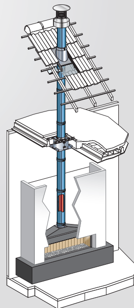
Ortakinis-dūmtakinis dūmtraukis BI-GAS; prijungimas (BI-GAS)
